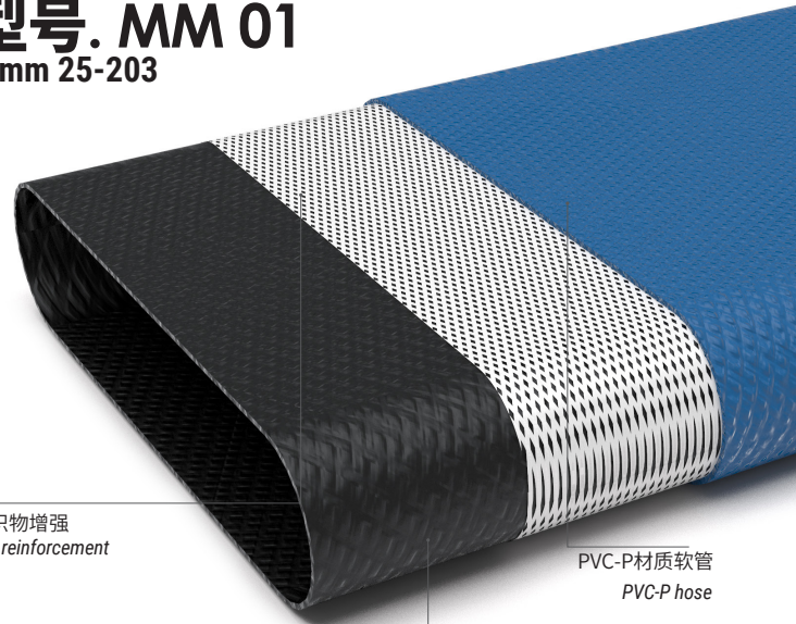
内胶材质PVC-NBR PVC-NBR liner
